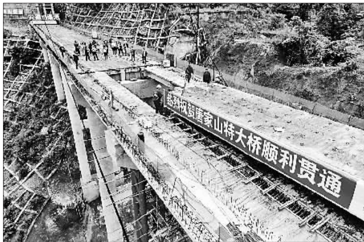
5月11日上午,随着四川北川羌族自治县唐家山堰塞湖跨湖大桥最后一块桥面梁架架完成,唐家山特大桥梁顺利贯通,预计今年8月底具备通行能力。 蒲滔摄/光明图片
